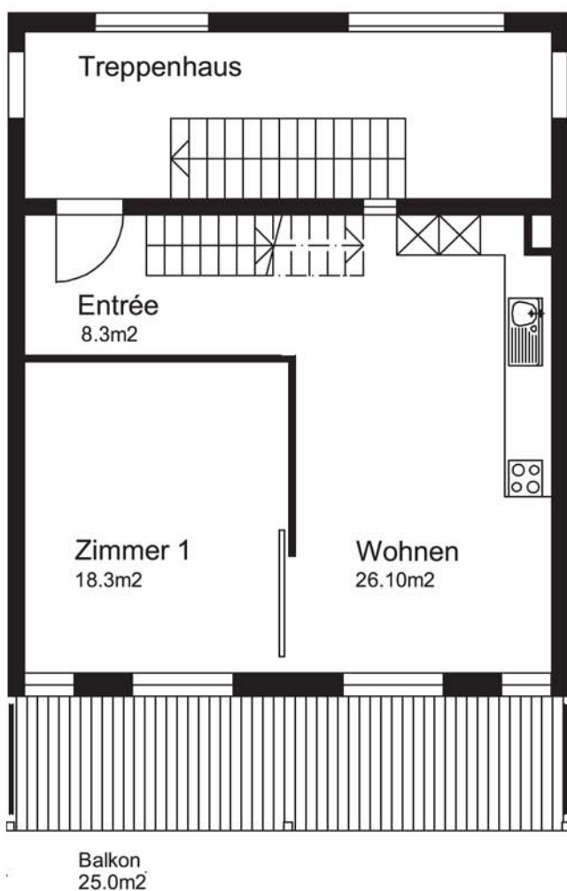
2. Obergeschoss
